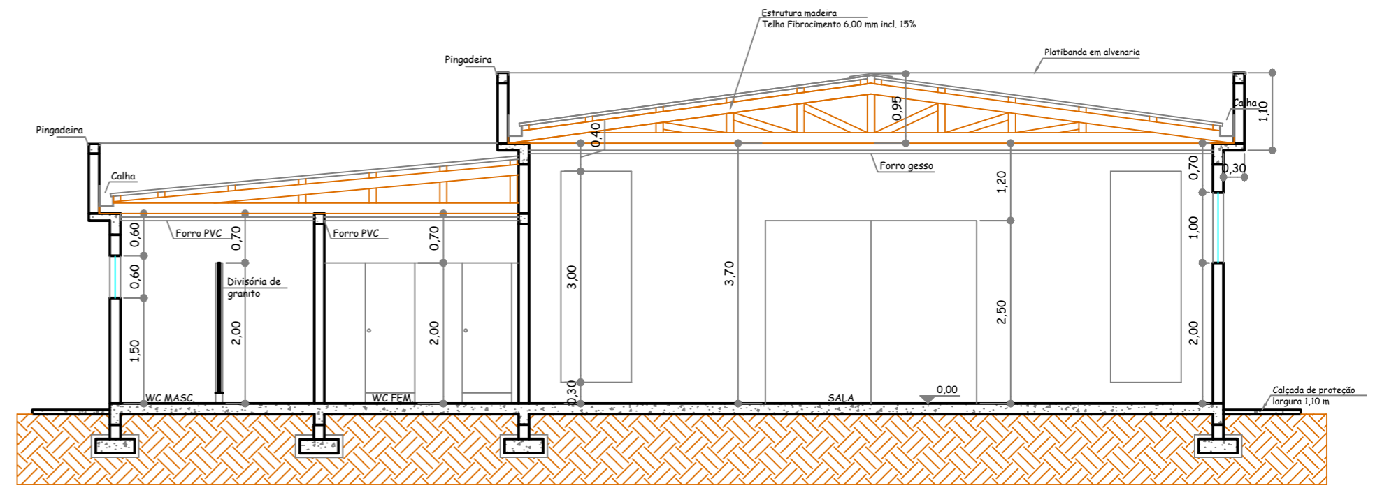
Corte A/B Escala 1:75
