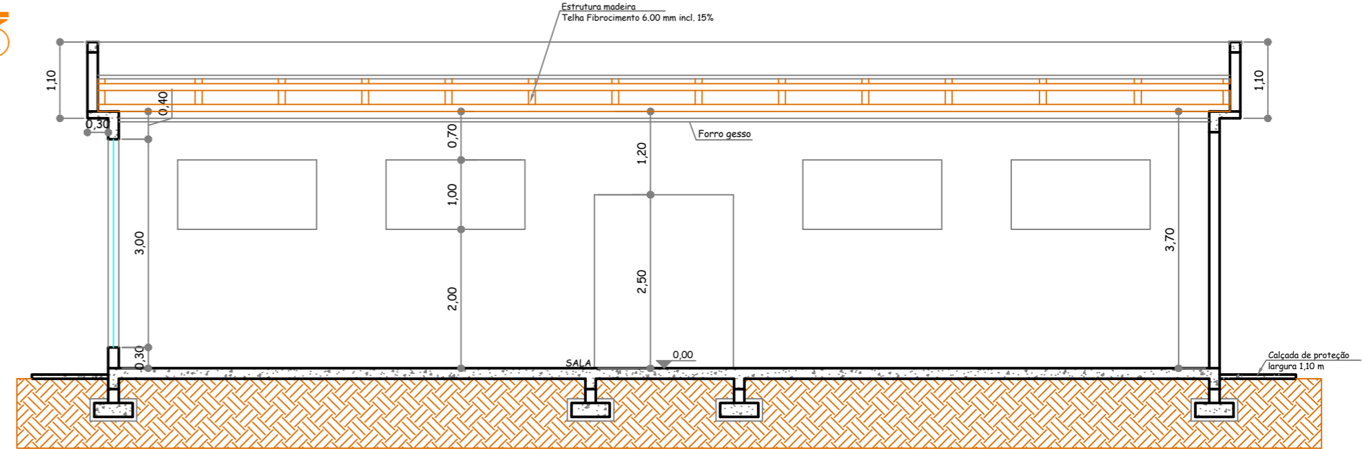
Corte C/D Escala 1:75
